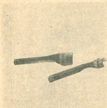
9. kép. Körvéső a lefolyó csatorna behelyezéséhez. A felsőbe beleszorítva a kb. 5×4 cm-nyi bádogcsatorna. (Term. nagyság \frac{1}{6} -része.)
