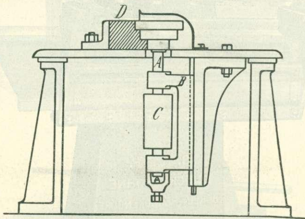
128. ábra. Marógép szerkezeti rajza.
