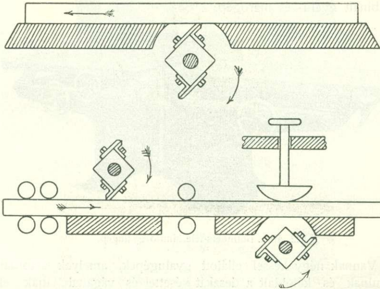
121. ábra. Gyaluszerszám elrendezése. I. A tárgy alatt. II. Alatta és fölötte.
