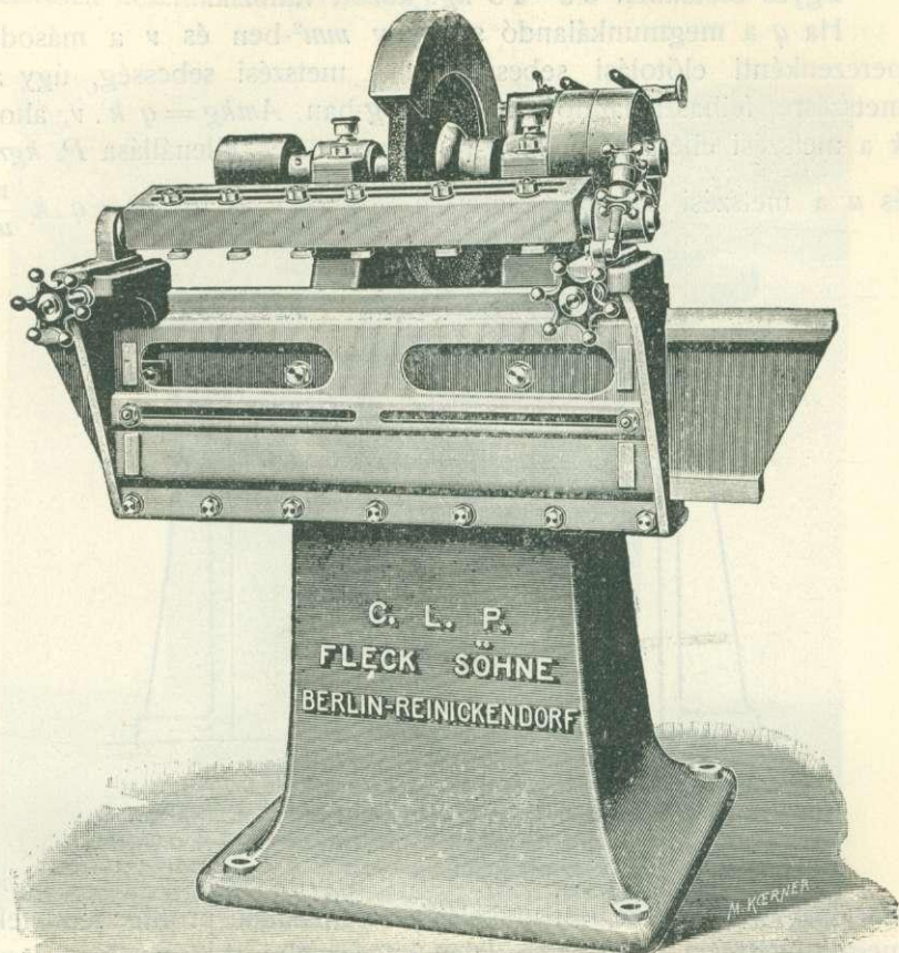
127. ábra. Gyalukés-köszörülő.
