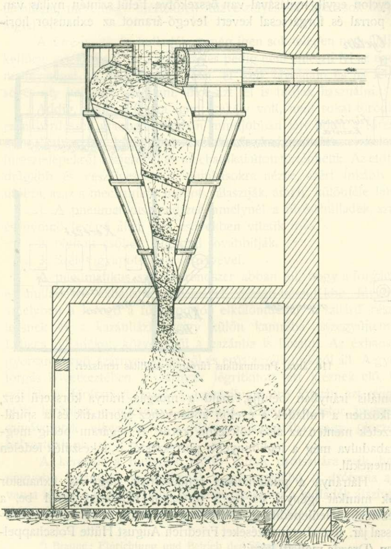
117. ábra. A ciklon szerkezete.
