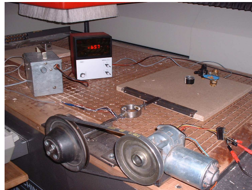
1. ábra – Vonszoló szerkezet az erőmérő cellával
