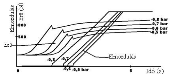
2. ábra – Erő és elmozdulás regisztrátum forgácslapnál
